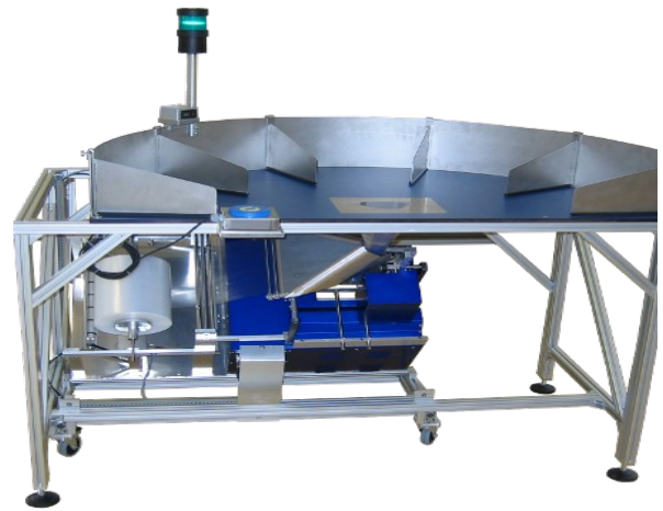
Abbildung 2: LBX100 Sortiertisch mit Einwurfföffnung in eine Lauper LVX Verpackungsmaschine (Anordnung unter dem Tisch)
