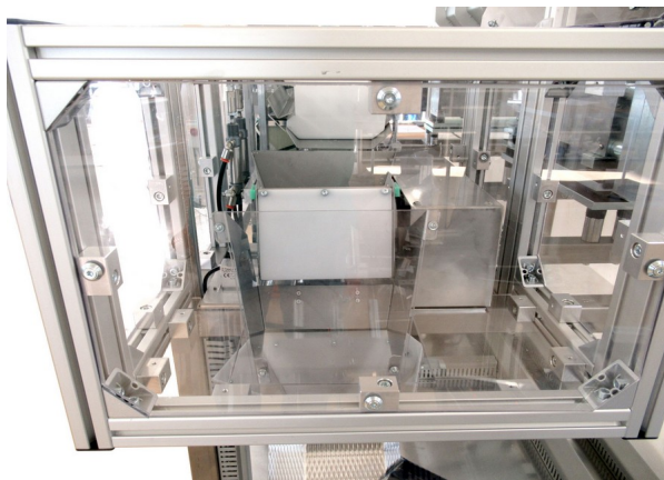
Abbildung 5: Der Wiegebehälter ist mit einem Gehäuse vor äusseren Einflüssen geschützt. Dies hat zu Folge, dass neben der Geräuschminderung die Zählgenauigkeit erhöht wird.
