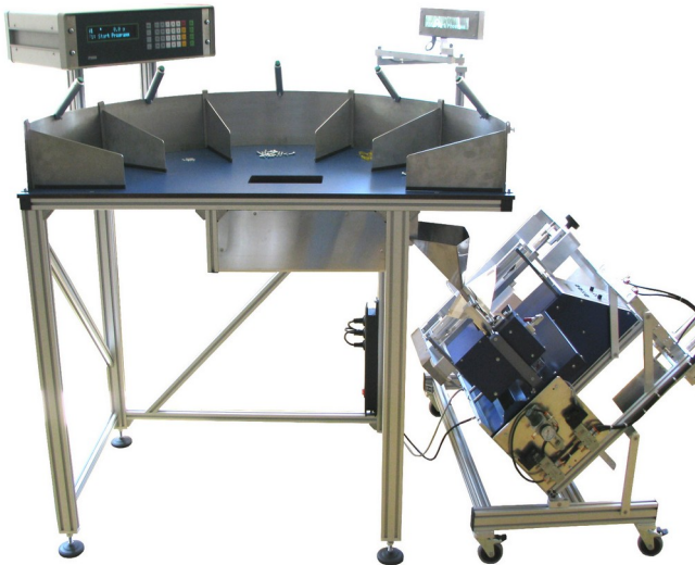
Abbildung 1: LT100 Zähl- und Wiegetisch mit Anbindung einer Lauper LVX Verpackungsmaschine
