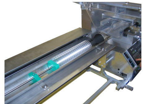
Abbildung 3: Anwendungsbeispiel Becherstapel-Verpackung mit rundem Einschiebe-Kanal
